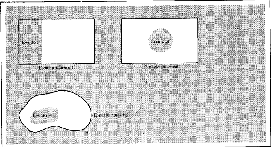
FIGURA 3.2 Algunos ejemplos de diagramas de Venn.
